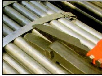
② 刃先の差込み
